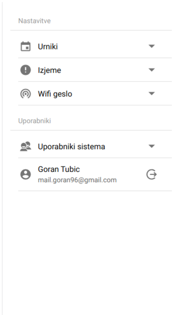
Slika 2: Nastavitveno okno
